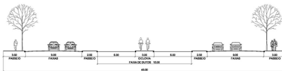
V 3.15 - Perfil especial da Av. Açucena no trecho entre a Av. Santos Ferreira e a Rua Boqueirão
