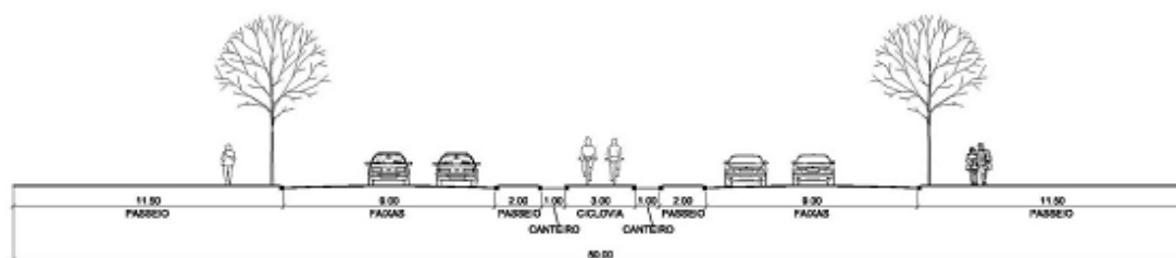
V 3.16 - Perfil da Rua Eng. Irineu Carvalho Braga
