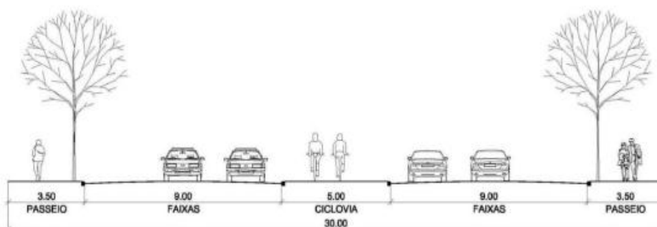
V 2.2 - Via Perimetral Perfil Básico com ciclovia
