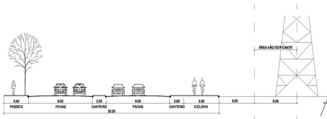
V 3.11 - Perfil especial da faixa de domínio da rede de energia elétrica da AES SUL
