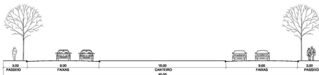
V 4.13 - Perfil da Av. Inconfidência no trecho do Loteamento Cidade Nova
