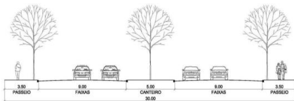
V 2.1 - Via Perimetral Perfil Básico
