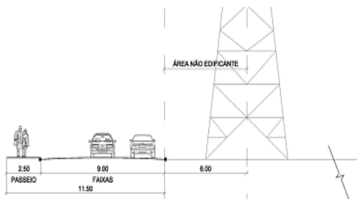
V 4.2 - Perfil especial junto à faixa de domínio da rede de energia elétrica da AES SUL no prolongamento da Rua 2 no Loteamento 103 há
