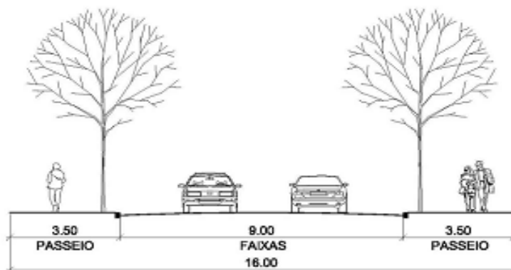
V 3.4 - Perfil da Av. Rio Grande do Sul ao redor das praças
