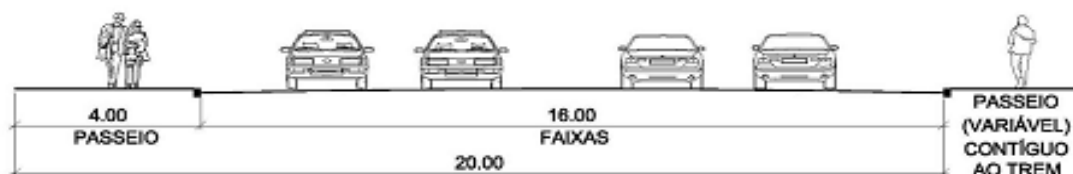
V.3.6 - Perfil da Av. Guilherme Schell
