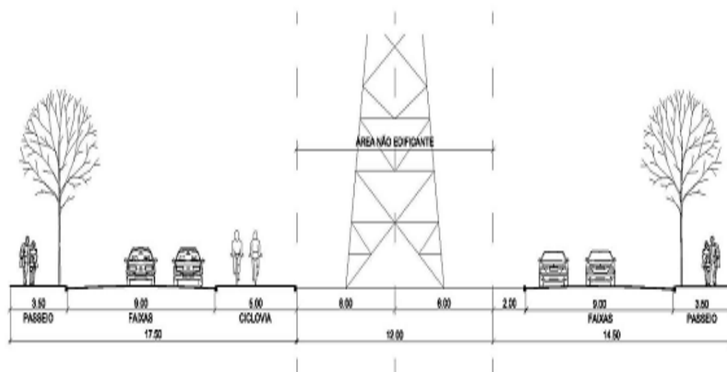
V 2.4 - Perfil especial da faixa de domínio da rede de energia elétrica da AES SUL junto ao Pólo Logístico
