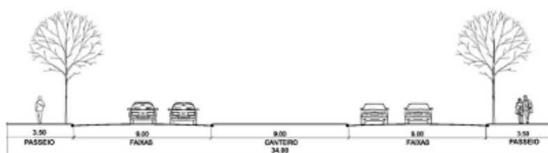
V 3.14 - Perfil especial da Rua República no trecho entre a Rua José Veríssimo e a Rua Curitiba
