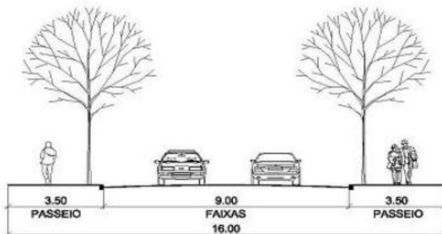
V 5.1 - Via Local Perfil Básico
