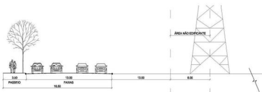
V 4.7 - Perfil especial junto à faixa de domínio da rede de energia elétrica da ELETROSUL
