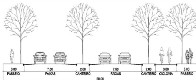
V 3.10 - Perfil especial da Av. das Canoas no trecho entre a BR 448 e a Praia de Paquetá
