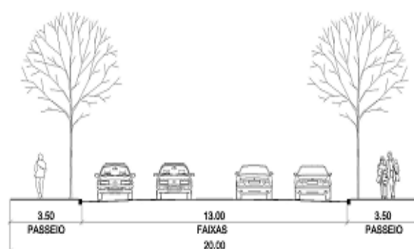
V 4.1 - Via Coletora Perfil Básico
