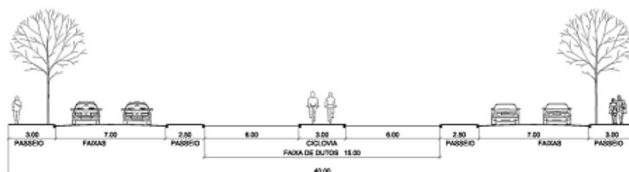
V 3.13 - Perfil especial da Rua Itamar Matos / Esperança junto ao Distrito Jorge Lanner
