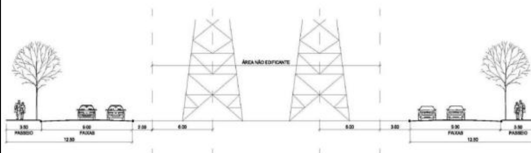
V 2.3 - Perfil especial da faixa de domínio da rede de energia elétrica da AES SUL junto a ETA
