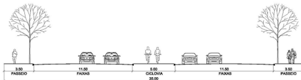
V 4.12 - Perfil da Av. Inconfidência no trecho entre BR 116 e o Loteamento Cidade Nova
