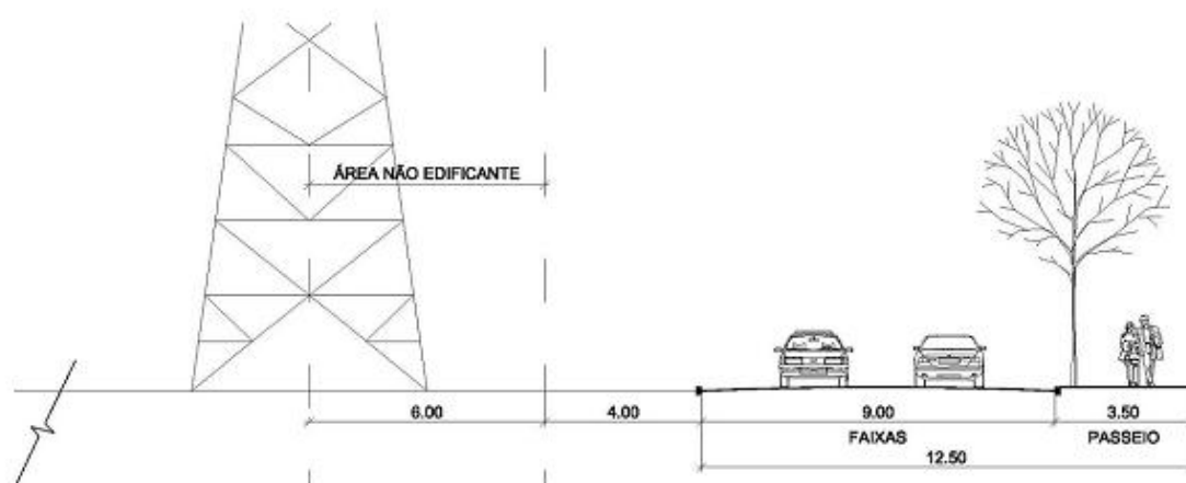
V 4.4 - Perfil especial junto à faixa de domínio da rede de energia elétrica da AES SUL próximo a ULBRA
