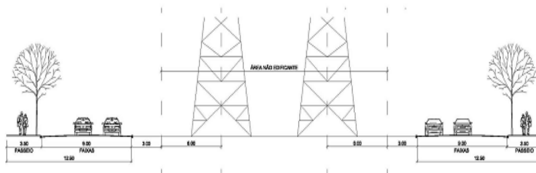
V 4.3 - Perfil especial junto à faixa de domínio da rede de energia elétrica da AES SUL no Loteamento 103 ha
