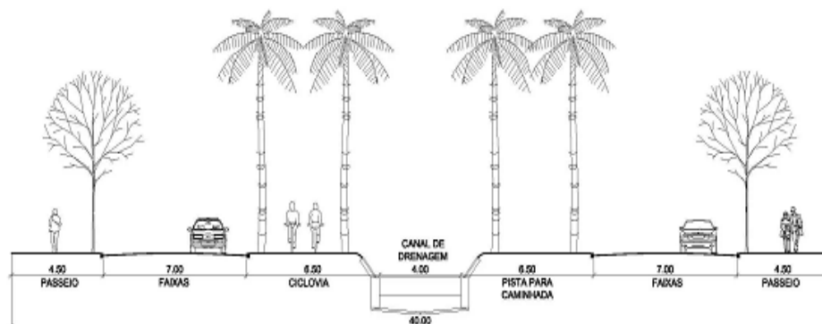
V 3.12 - Perfil especial da Av. das Canoas no trecho entre a Avenida A e a BR 448
