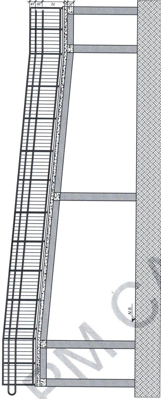
CORTE AA Esc: 1/50
