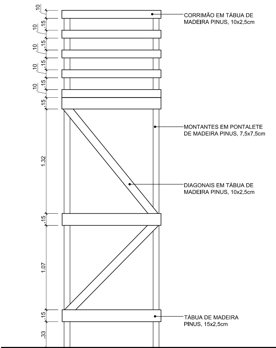
ELEVAÇÃO 01 | ESCADA PROVISÓRIA escala 1:25
