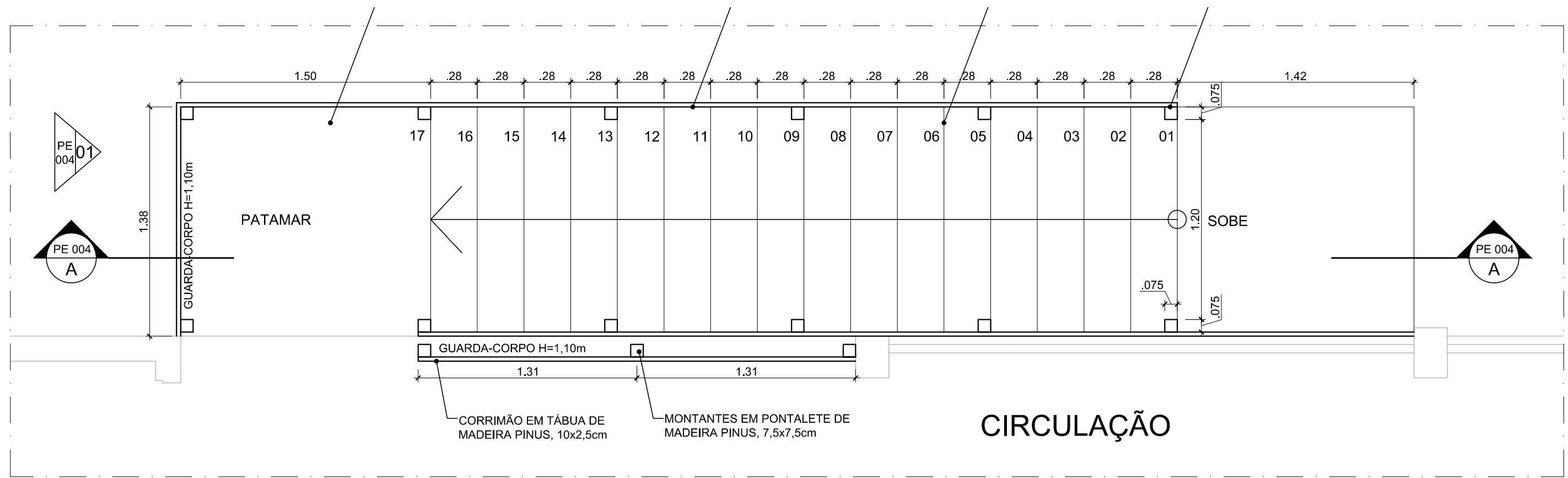
■ PLANTA BAIXA | ESCADA PROVISÓRIA escala 1:25
