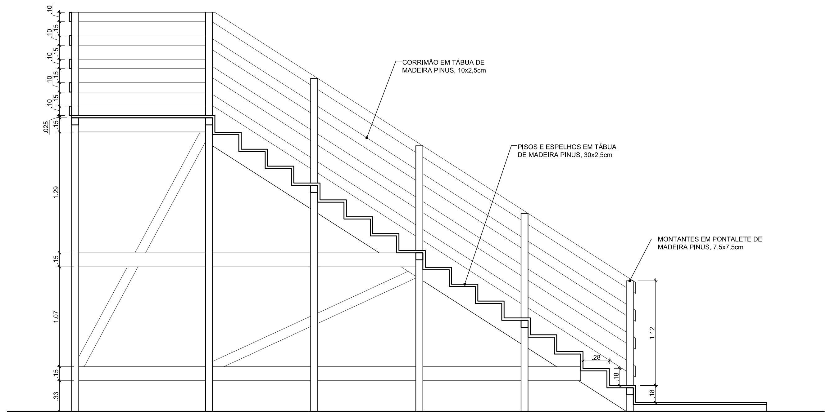
CORTE A | ESCADA PROVISÓRIA escala 1:25
