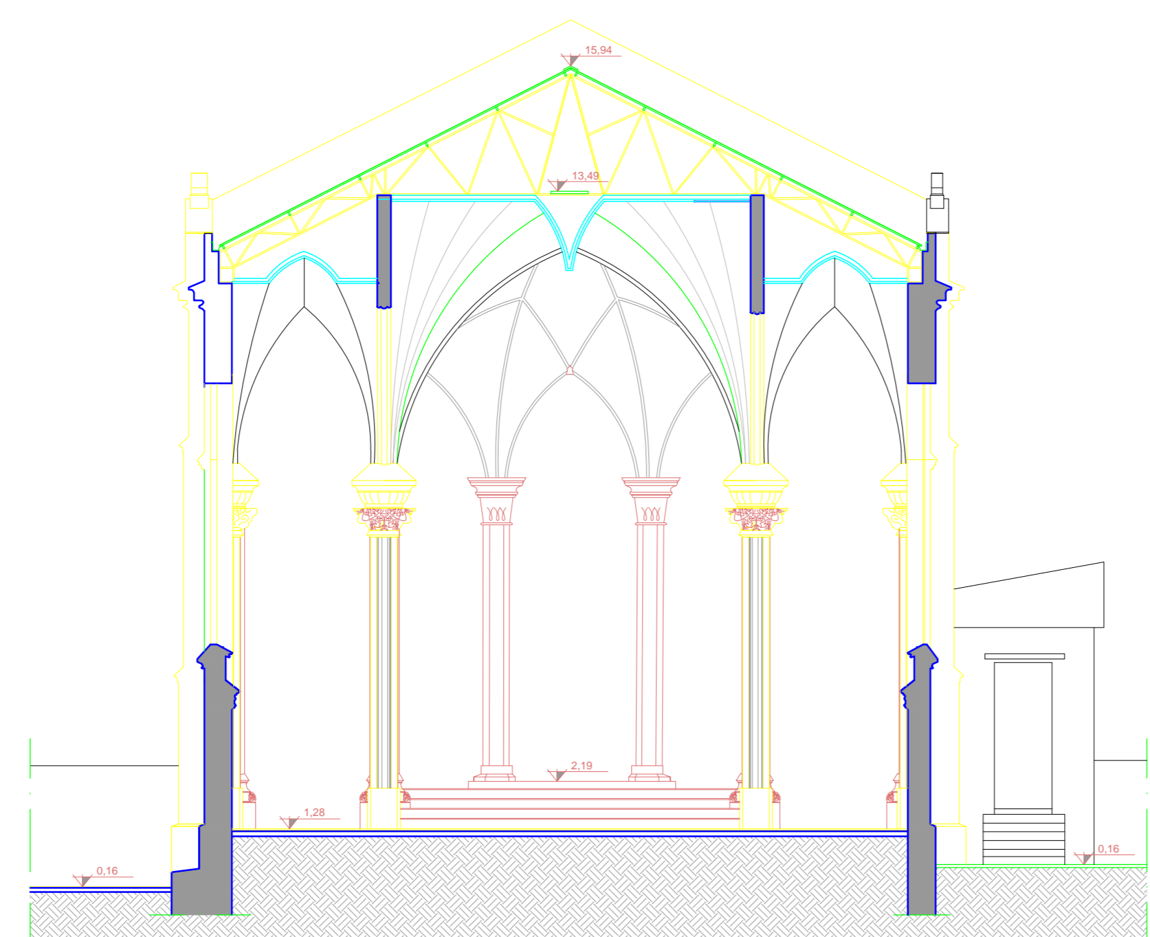
CORTE TRANSVERSAL B-B ESCALA 1/75
