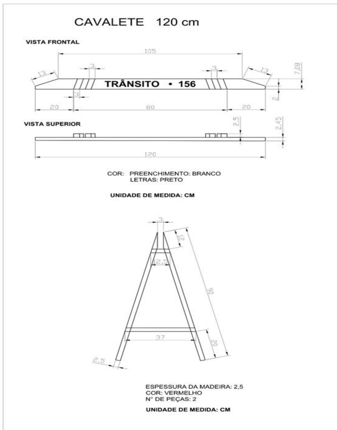
MODELO DE CAVALETE DE MADEIRA
