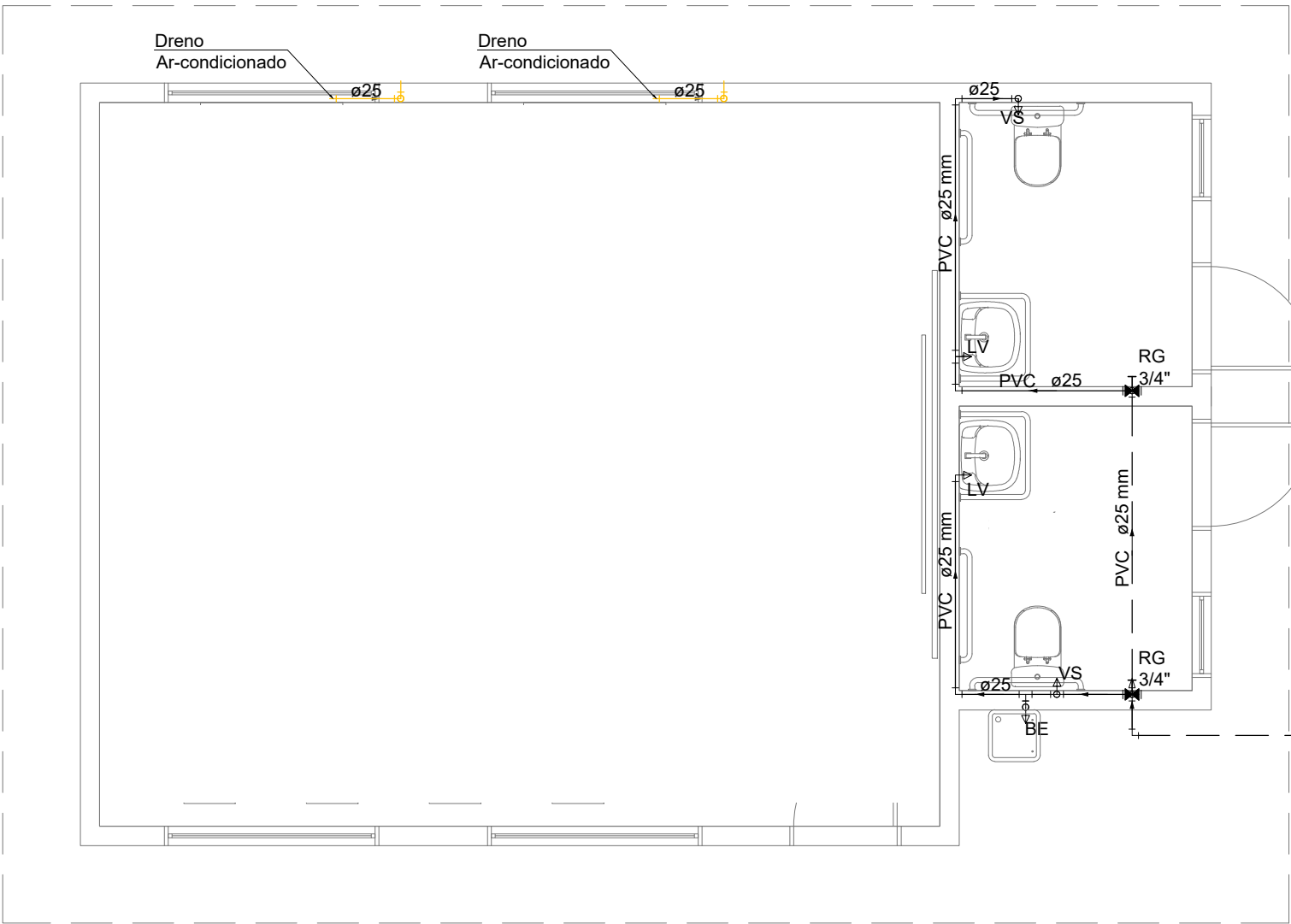
PLANTA BAIXA - ÁGUA FRIA ESCALA 1:50
