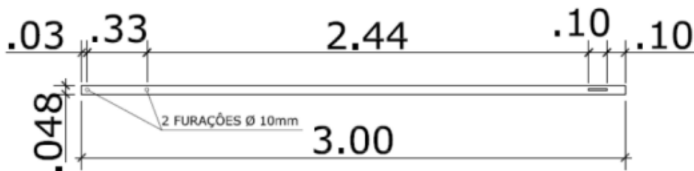
VISTA LATERAL
